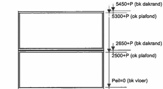
Doorsnede A-A
