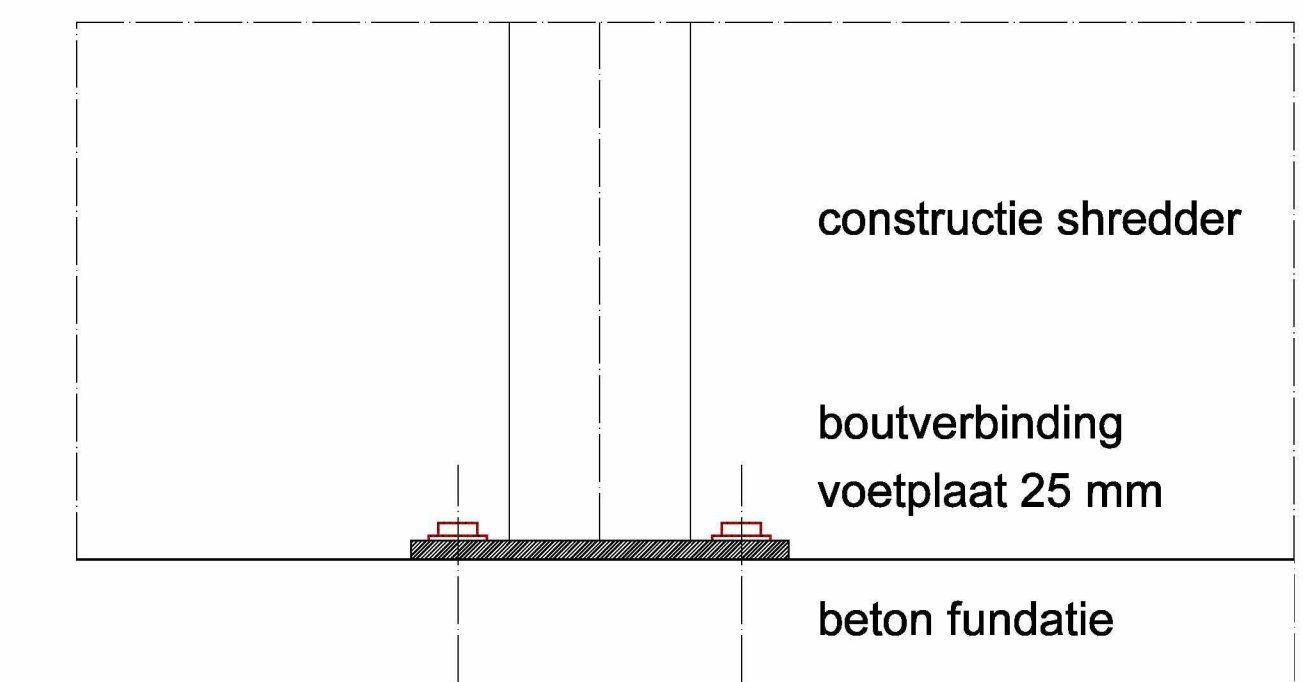
detail A / 1:10 bevestiging shredder op fundatie
